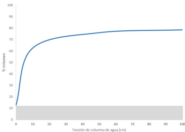
CURVA RETENCIÓN HÍDRICA CULTIVATOR
